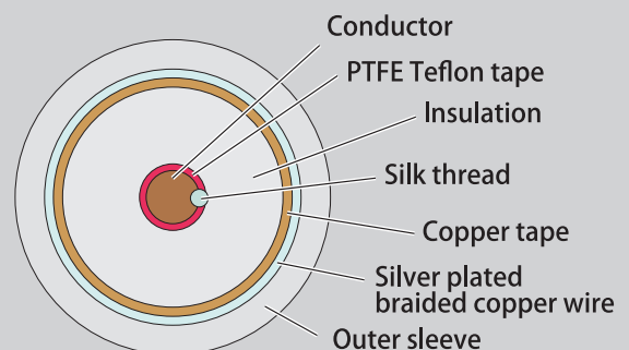
7N-D5050 Leggenda Cable structure
