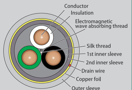
7N-PC4030 Leggenda Cable structure
